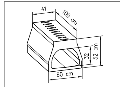
ACO PRO AT 500 geschlitzt
