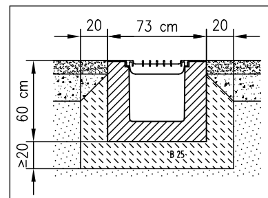
Einbau in wassergebundener Decke
