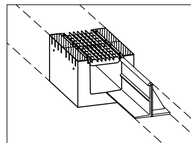
ACO PRO Stopprinne mit Leitwand
