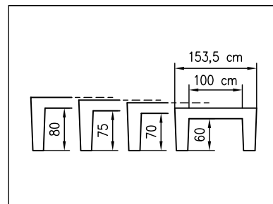
Bauhöhen ST 1000
