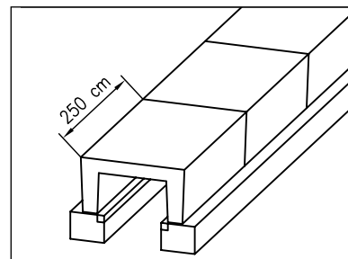
ST 1000 auf Streifenfundament
