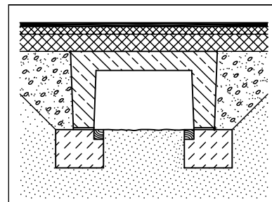
Einbausituation Asphaltfahrbahn
