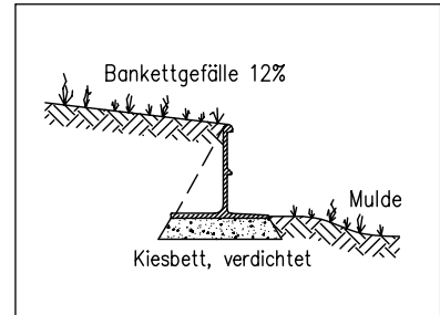
Einbau Bankett
