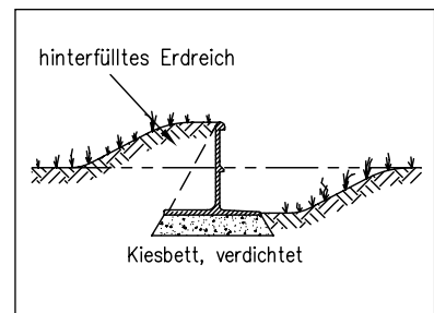
Einbau ebenes Gelände, vertieft
