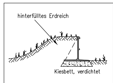
Einbau ebenes Gelände, angeschüttet
