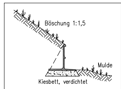
Einbau Böschung
