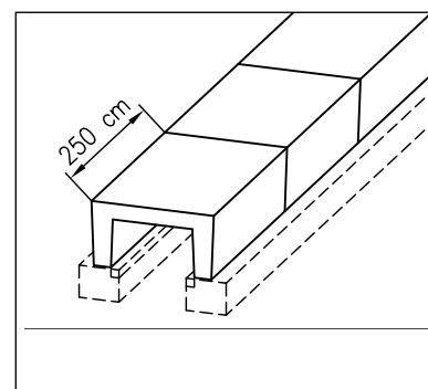
ST 1000 auf Streifenfundament
