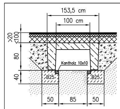
Einbausituation Asphaltfahrbahn
